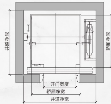
井道平面布置图
