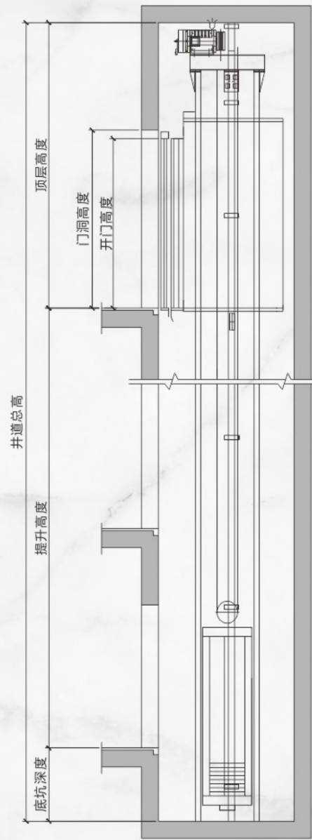
井道立面图
